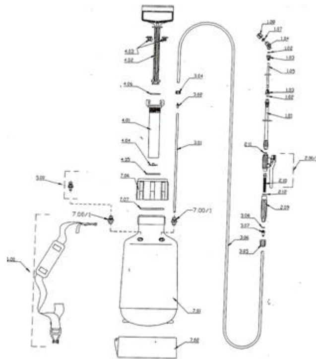
Schéma postřikovače Orion
